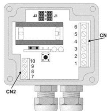
Abbildung 8 IP65 Modell
